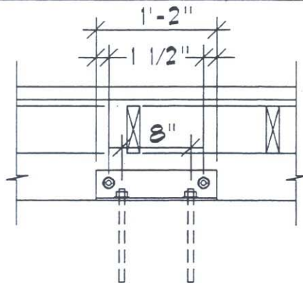
DETAIL 'B-B'
